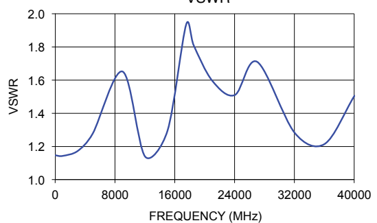
VSWR
