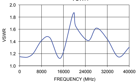
VSWR
