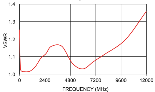
VSWR
