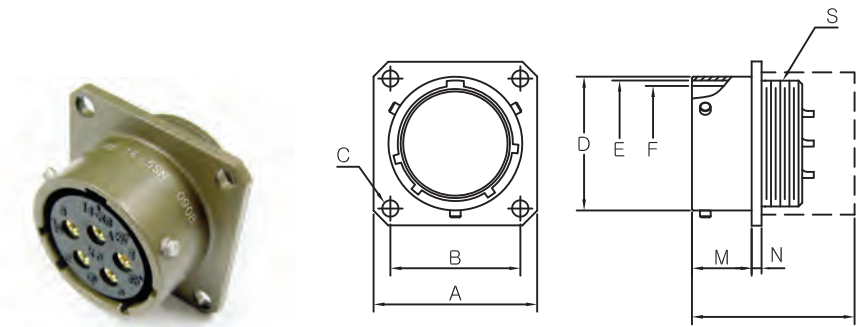
终端组件 Termination Assembly
